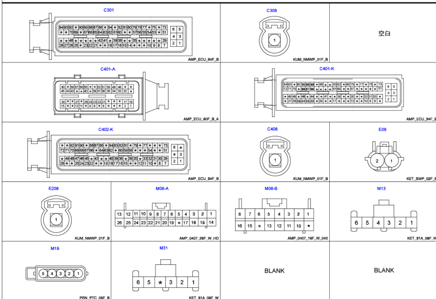
鼓风机 &amp; 空调控制系统( 自动) (6)
